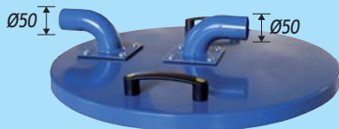
Vorabscheiderdeckel Ø 590
